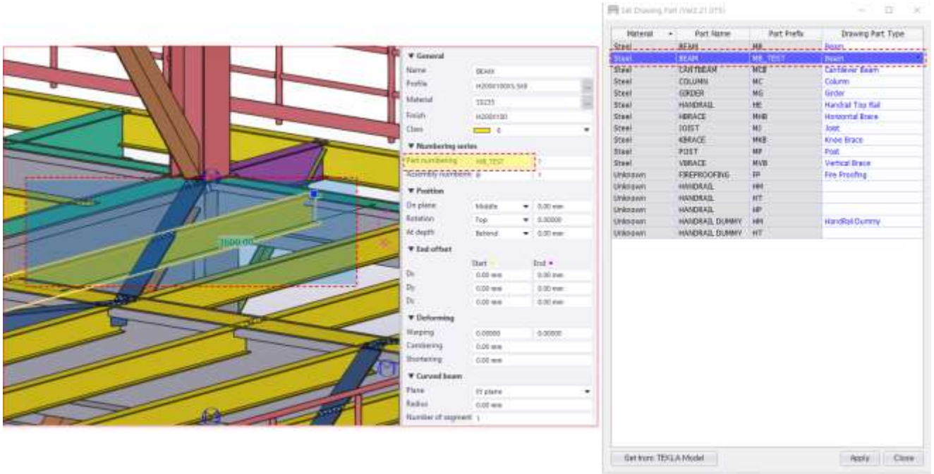
[ 모델에서 작성된 부재 정보 & Set Drawing Part 정의 ]
