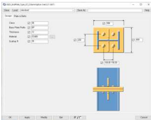
[ "End Plate Type의 Column Splice Connection" 화면 ]
